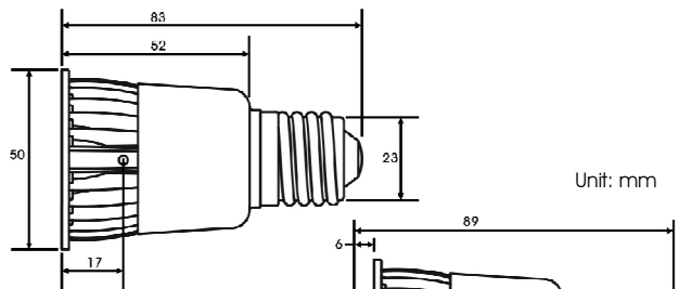
TRISTAR-E27
